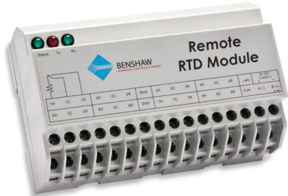
Optional RTD modules
